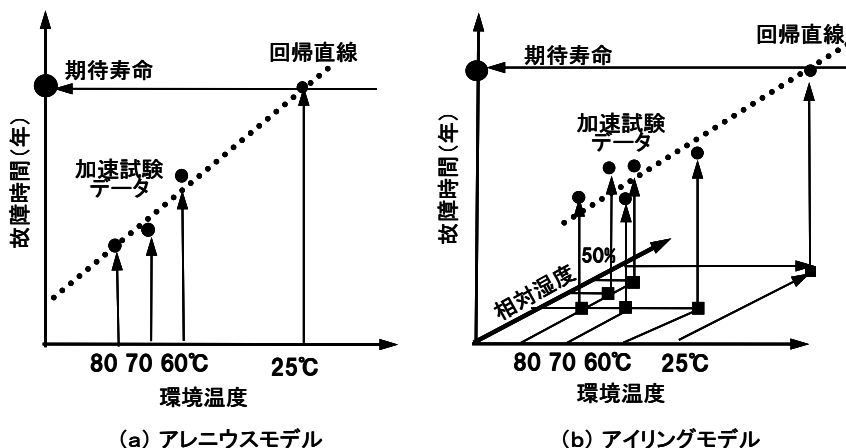
図2 加速試験による寿命推定の概略図
