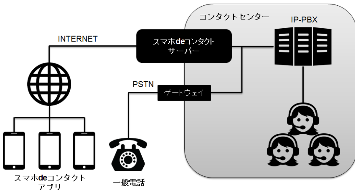
図.2 「スマホdeコンタクト」を用いたネットワーク構成図例
