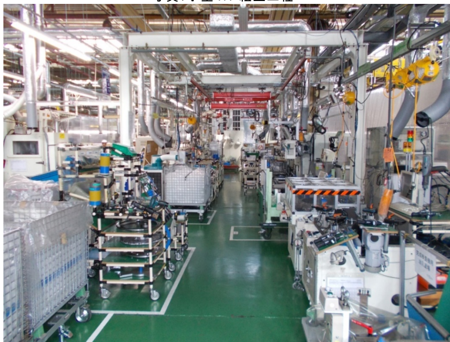
写真: 小型 HV 組立工程
