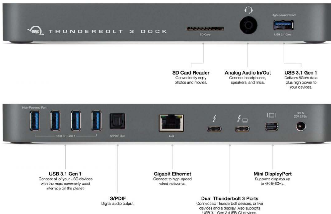
<写真 OWC 12ポート Thunderbolt 3 Dock (ドック) ポート配置>
