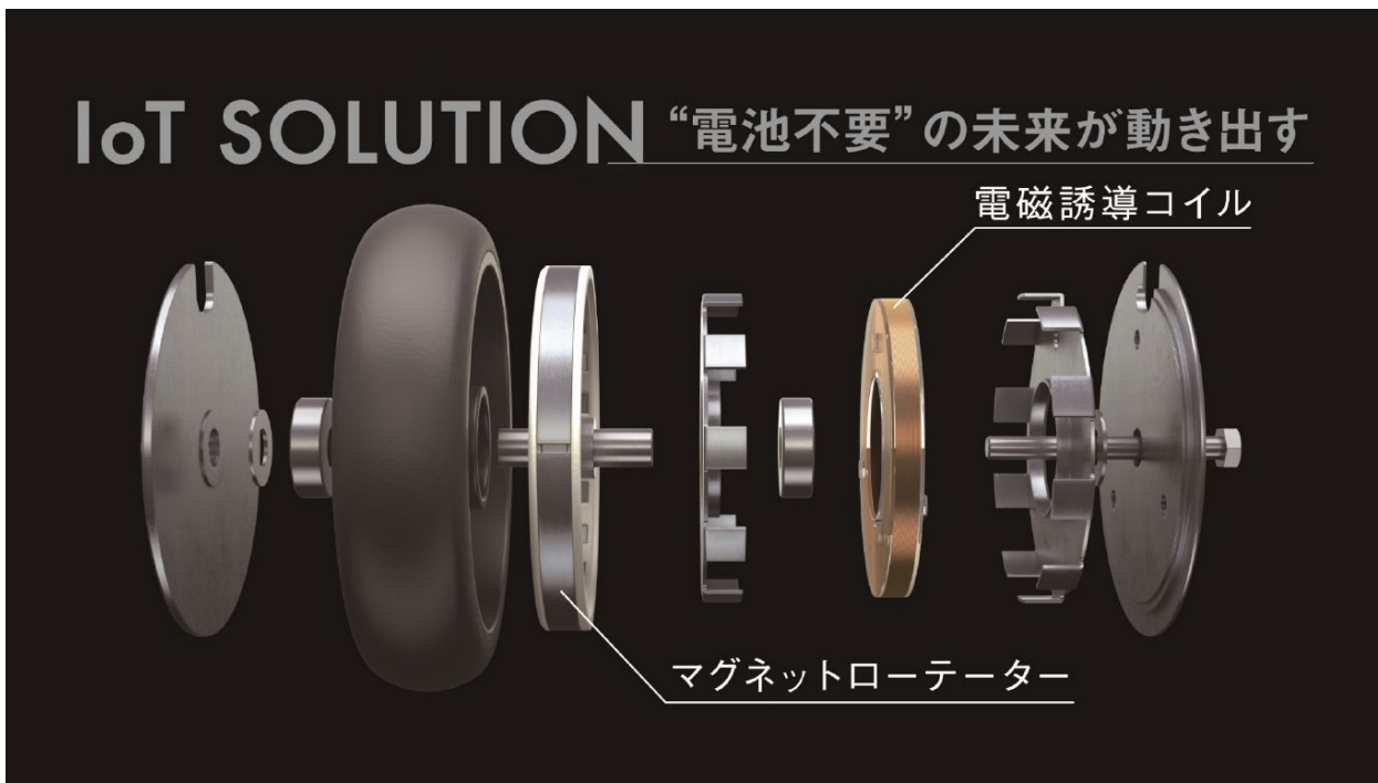
■スマートキャスターの発電構造イメージ
